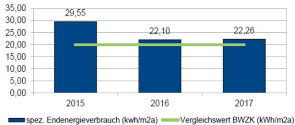
Stromverbrauch der Liegenschaft 2015 bis 2017
